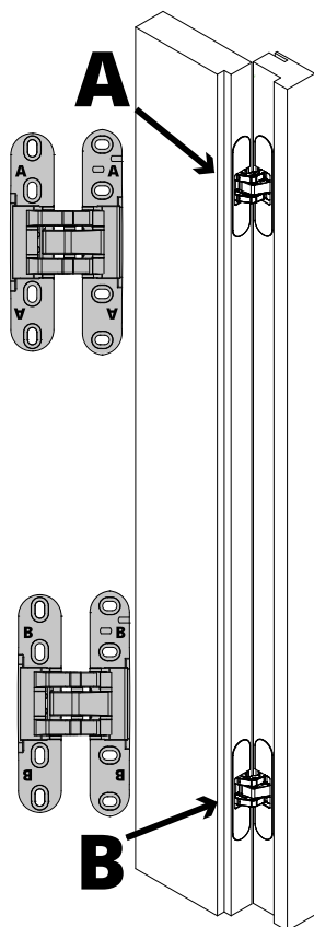
Fraisage côté ouvrant
