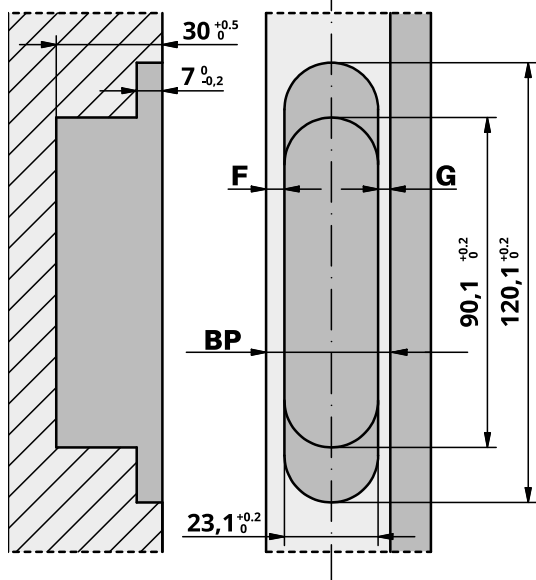
Fraisage côté ouvrant
