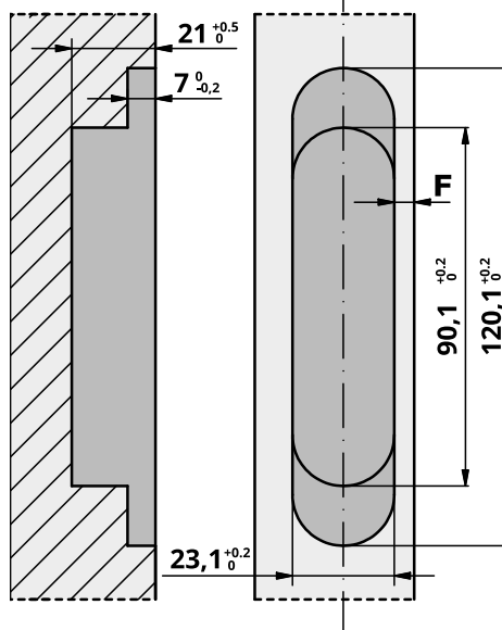
Fraisage côté dormant
