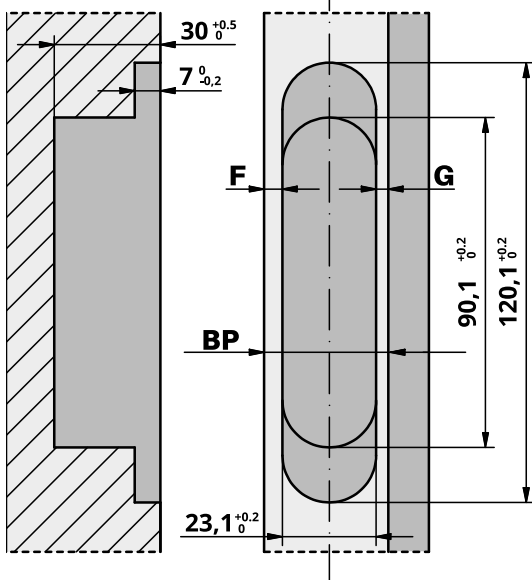
Ausfräsung Tür-Seite
