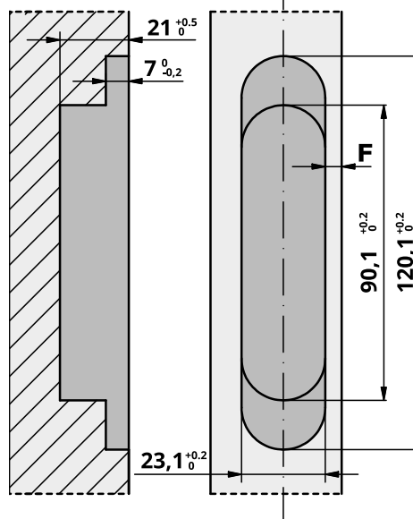
Ausfräsung Rahmen-Seite
