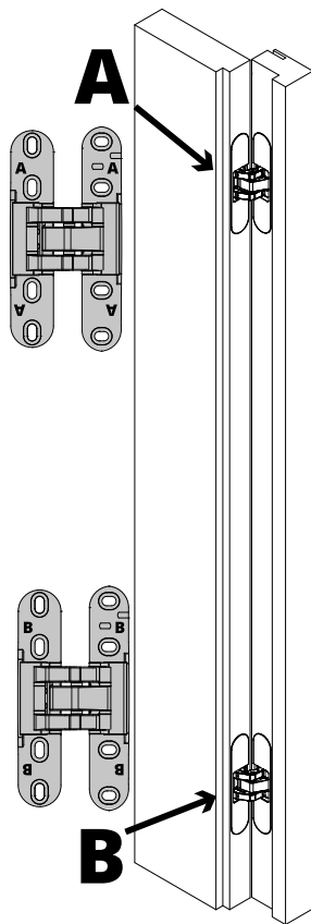
Ausfräsung Tür-Seite
