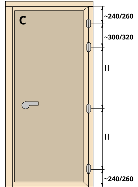
4 hinges
