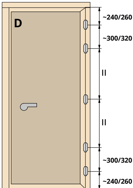
5 hinges
