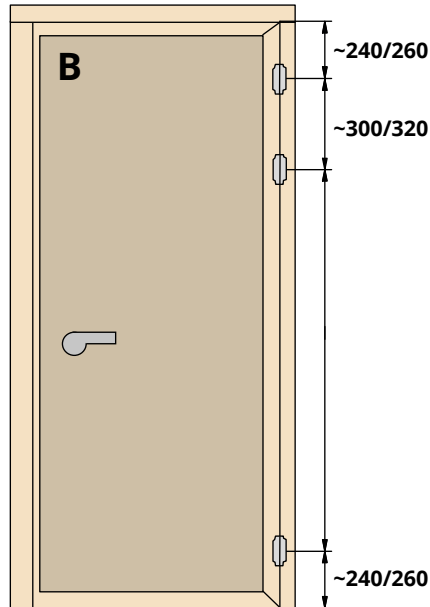
3 hinges
