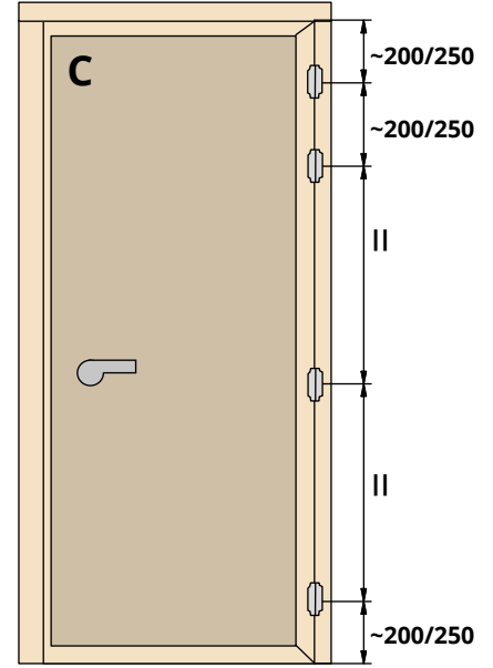
Cuatro bisagras
